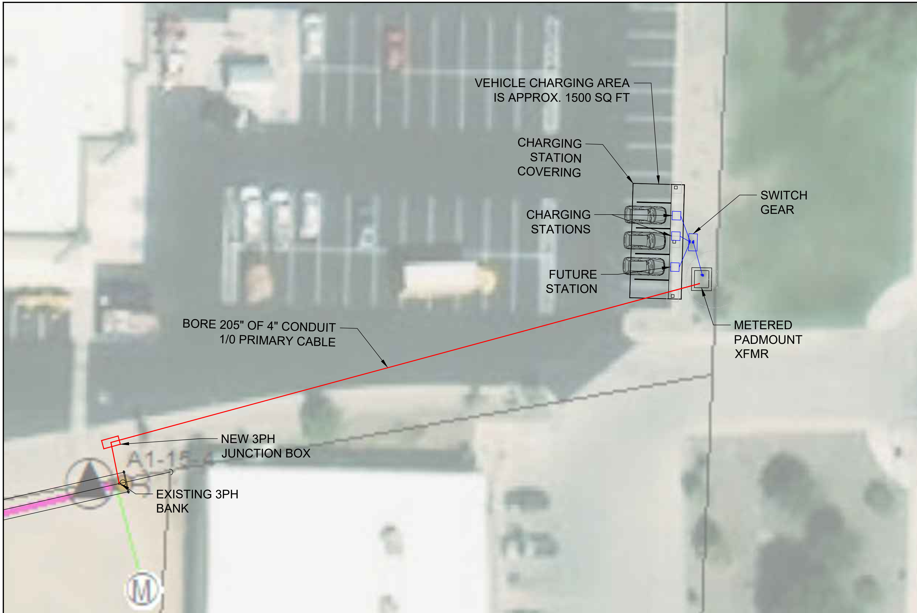
PLAN VIEW SCALE: 1/8" = 1'0"
